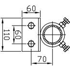
Schnitt E-F Schnitt A-B
