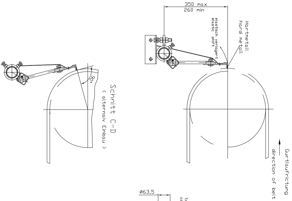
Schnitt C-D
